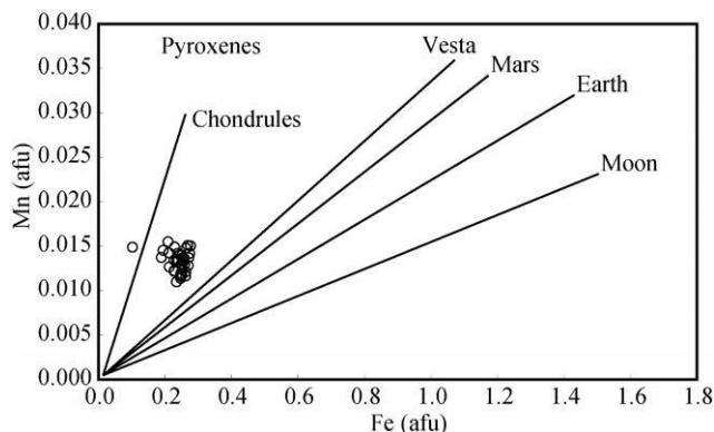
图 10 GRV 052382 陨石的易变辉石的 Mn-Fe 关系图
