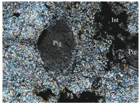
图 3 陨石内部结构
