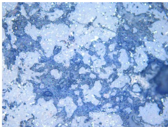
图6 富碳质不透明暗色区结构
