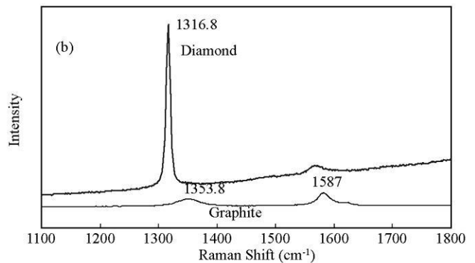
图 7 石墨中金刚石颗粒二次电子图像 (a)和金刚石及石墨的激光拉曼光谱 (b)
