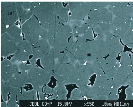
图 4 橄榄石细晶结构的背散射电子图片
