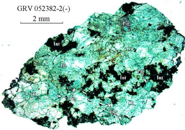
图 2 GRV 052382-2薄片显微照相全貌拼图
